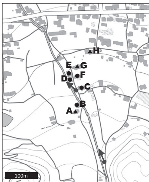
図50 久留米市田主丸町竹野の被災場所周辺図。図中矢印は写真12、写真13の撮影位置と方向。●：建物が全部倒壊・流失，▲：建物の一部が倒壊
