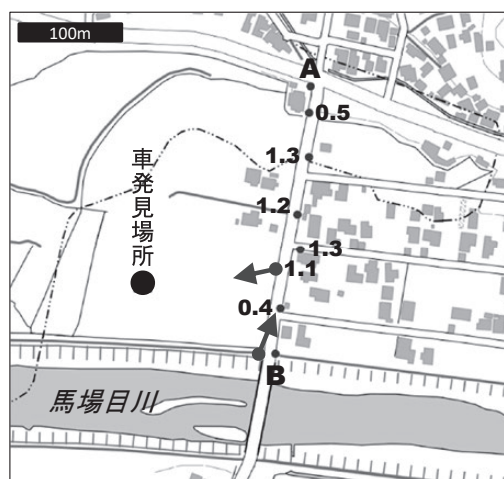
図62 五城目町大川西野の被災場所周辺図。図中矢印は写真17、写真18の撮影位置と方向。数字は現地で計測した道路面からの浸水深
