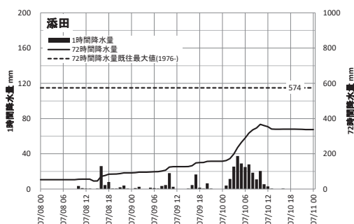
図43 AMeDAS 添田の降水量（2023年7月8日～10日）
