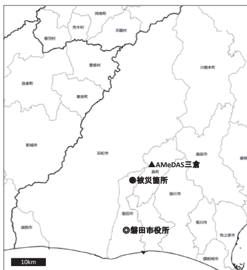
図1 磐田市大平の位置略図。地理院地図（白地図）に加筆，上側が北，以下同様
