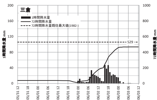
図3 AMeDAS 三倉の降水量（2023年5月31日～6月3日）
