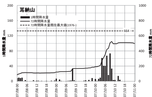
図51 AMeDAS 耳納山の降水量(2023年7月8日～10日)
