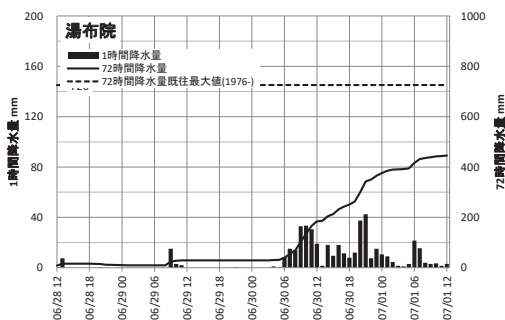
図23 AMeDAS 湯布院の降水量（2023年6月28日～7月1日）
