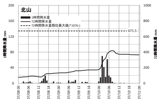
図47 AMeDAS 北山の降水量 (2023年7月8日～10日)
